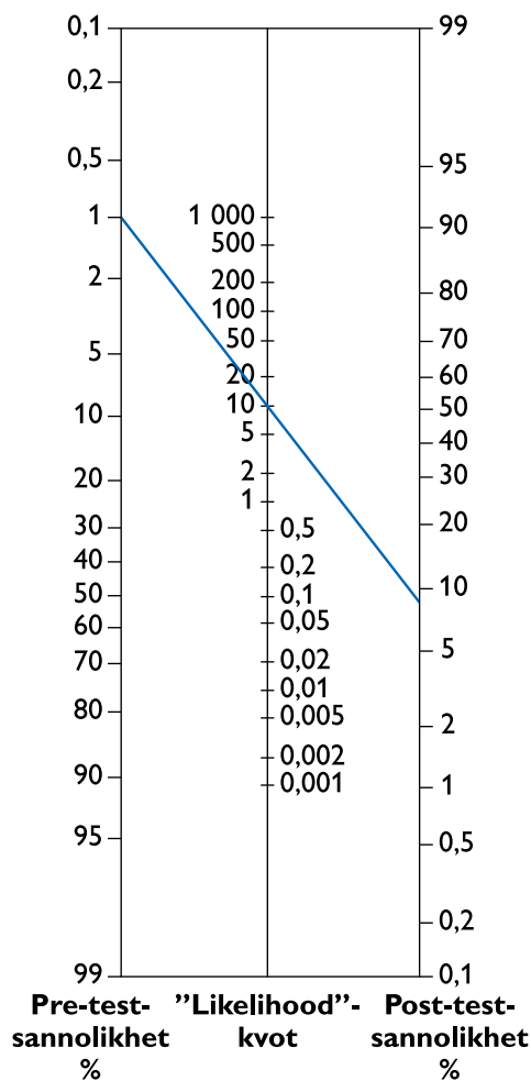
Figur B9.4 Nomogram.
