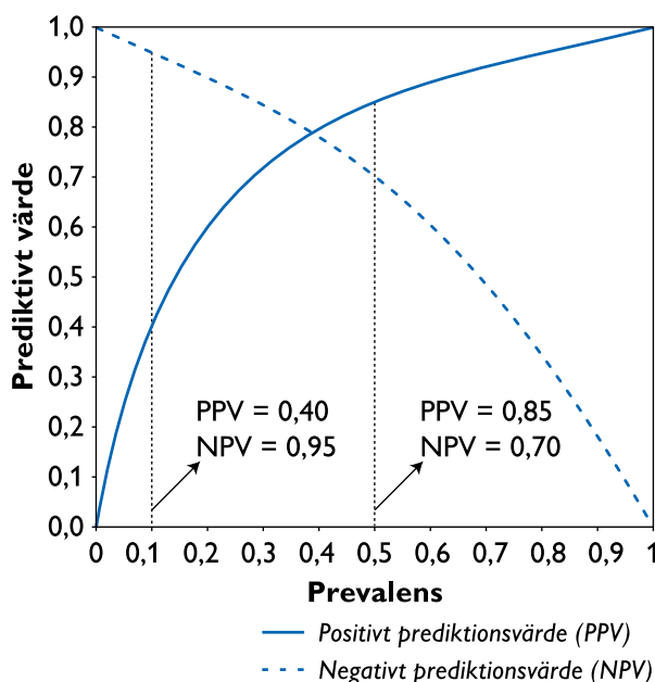
Figur B9.3 Diagram som illustrerar hur det positiva och negativa prediktionsvärdet påverkas av sjukdomsprevalensen. I exemplet är sensitiviteten (andelen sanna positiva) 0,6 och specificiteten (andelen sanna negativa) 0,9. Vid en sjukdomsprevalens på 10 procent blir det positiva prediktiva värdet (PPV) 0,40 medan det negativa prediktiva värdet (NPV) är 0,95. Om sjukdomsprevalensen är 50 procent, ökar PPV till 0,85, medan NPV sjunker till 0,70.
