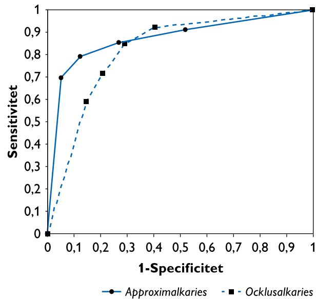
Figur B9.5 ROC-kurvor.
